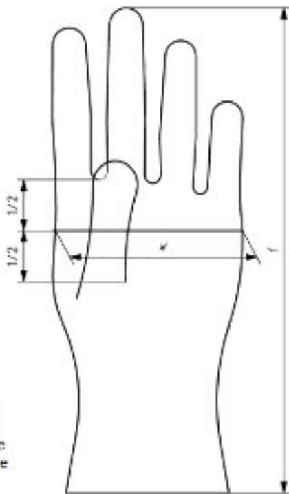
Bild 1 — Bestimmung der Länge und Breite von Handschuhen
